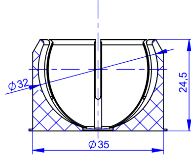
A-A KESİTİ
