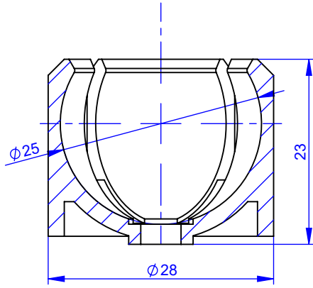
A-A KESİTİ
