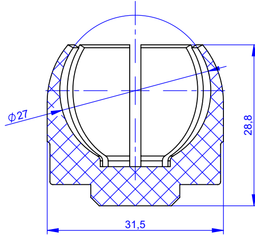
A-A KESİTİ
