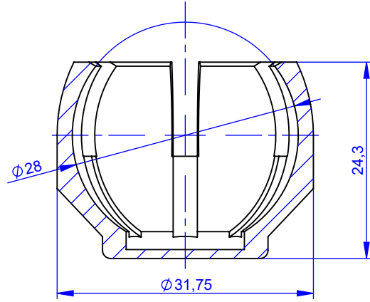
A-A KESİTİ
