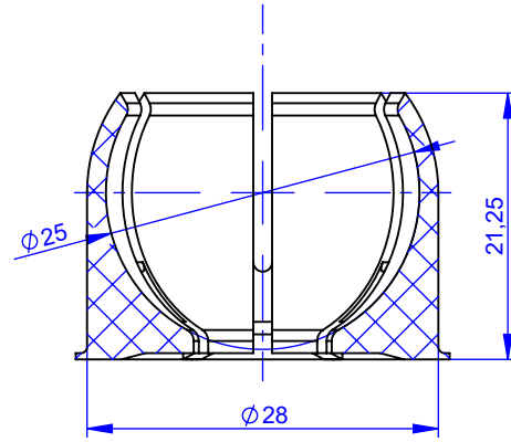
A-A KESİTİ
