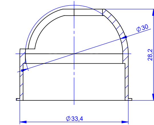
A-A KESİTİ
