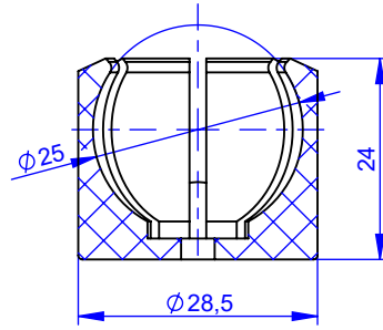
A-A KESİTİ
