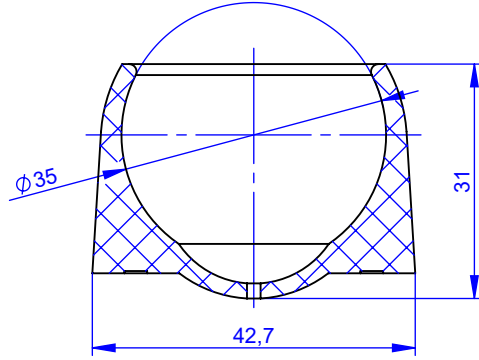
A-A KESİTİ
